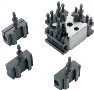
快換刀架
