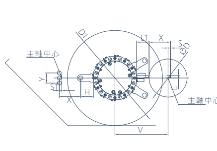
雙主軸 雙刀塔 Y軸 VDI徑向動力刀塔(選配) 單位:mm
