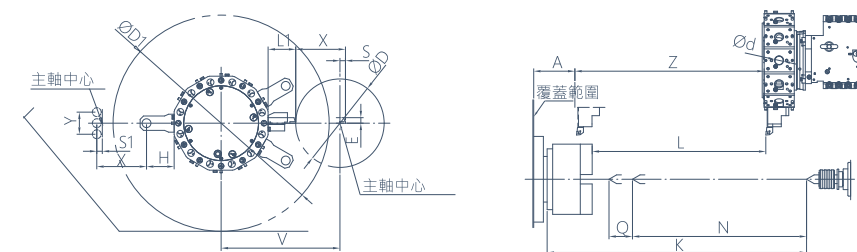
Y軸 VDI徑向動力刀塔(選配)
