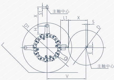
雙主軸 雙刀塔 VDI徑向動力刀塔(選配) 單位:mm
