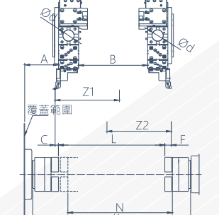
雙主軸 雙刀塔 Y軸 BMT徑向動力刀塔(選配) 單位:mm
