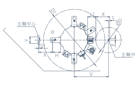
雙主軸 雙刀塔 Y軸 BMT徑向動力刀塔(選配) 單位:mm
