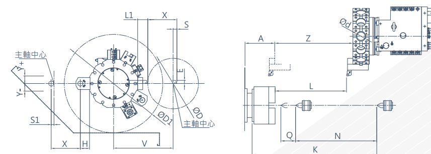
Y軸 BMT徑向動力刀塔(選配)
