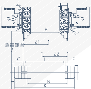
雙主軸 雙刀塔 VDI徑向動力刀塔(選配) 單位:mm
