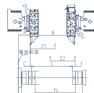
雙主軸 雙刀塔 Y軸 VDI徑向動力刀塔(選配) 單位:mm
