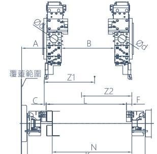
雙主軸 雙刀塔 BMT徑向動力刀塔(選配) 單位:mm
