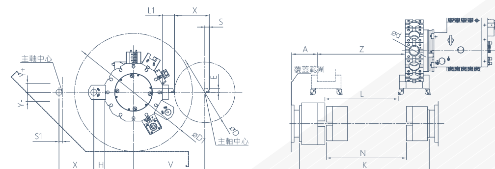
雙主軸 單刀塔 Y軸 BMT徑向動力刀塔(選配)
