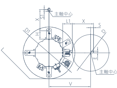
雙主軸 雙刀塔 BMT徑向動力刀塔(選配) 單位:mm
