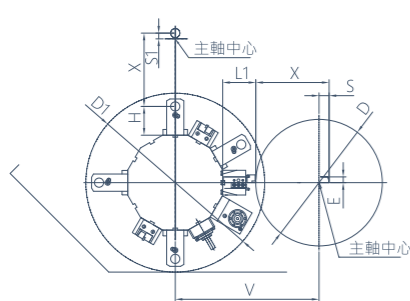
雙主軸 雙刀塔 BMT徑向動力刀塔(選配)
