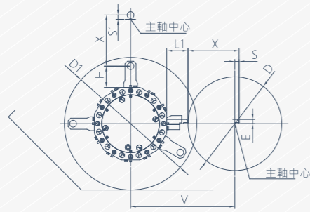
雙主軸 雙刀塔 VDI徑向動力刀塔(選配)
