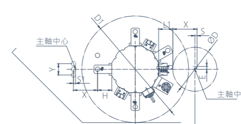
雙主軸 雙刀塔 Y軸 BMT徑向動力刀塔(選配)
