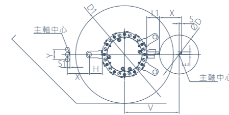
雙主軸 雙刀塔 Y軸 VDI徑向動力刀塔(選配)
