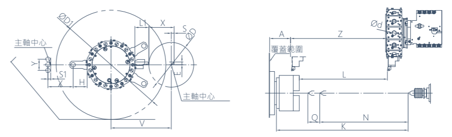
Y軸 VDI徑向動力刀塔(選配)
