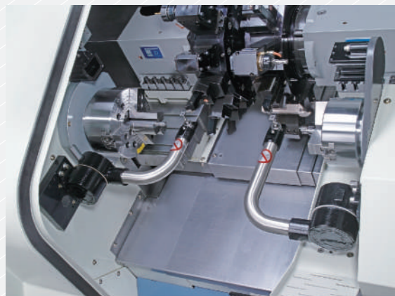
刀具測量系統 手動/自動擺臂 ESG (選配)
