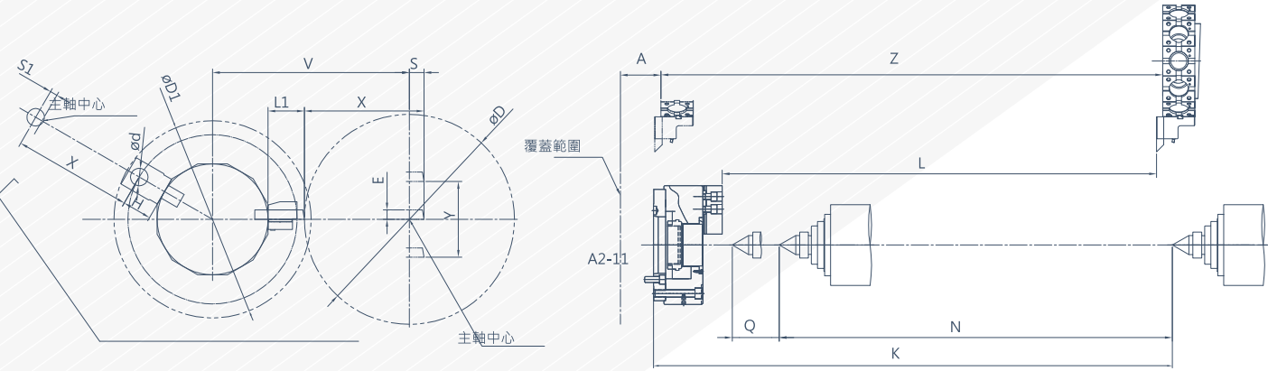
TC-Y軸 BMT動力刀塔 僅40/45/50系列 ( 選配 ) 單位:mm
