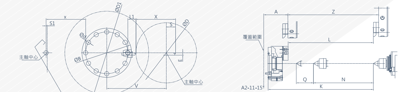
VDI軸向動力刀塔 ( 選配 ) TC-50L22 ~ TC-5072 單位:mm
