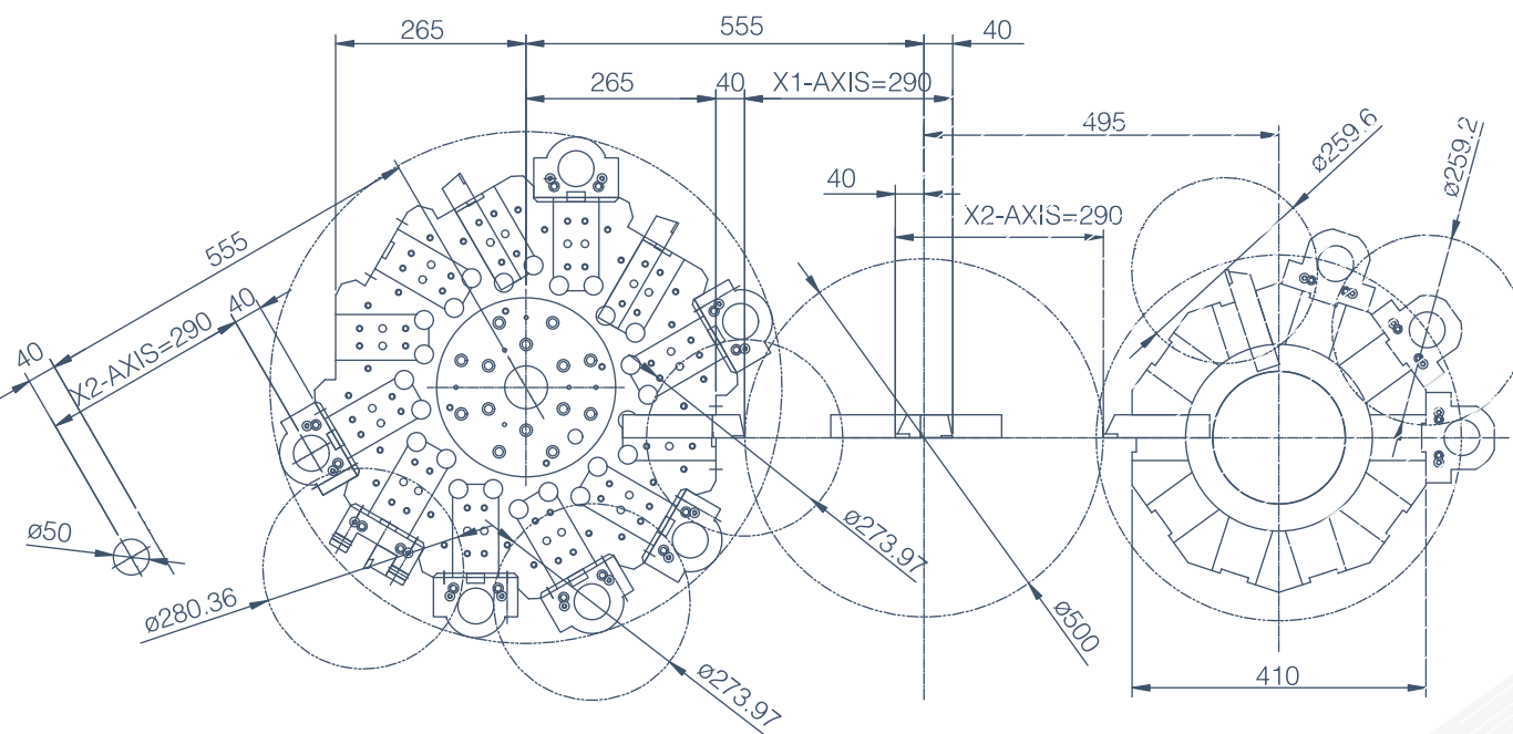
機型：TC-40T2
