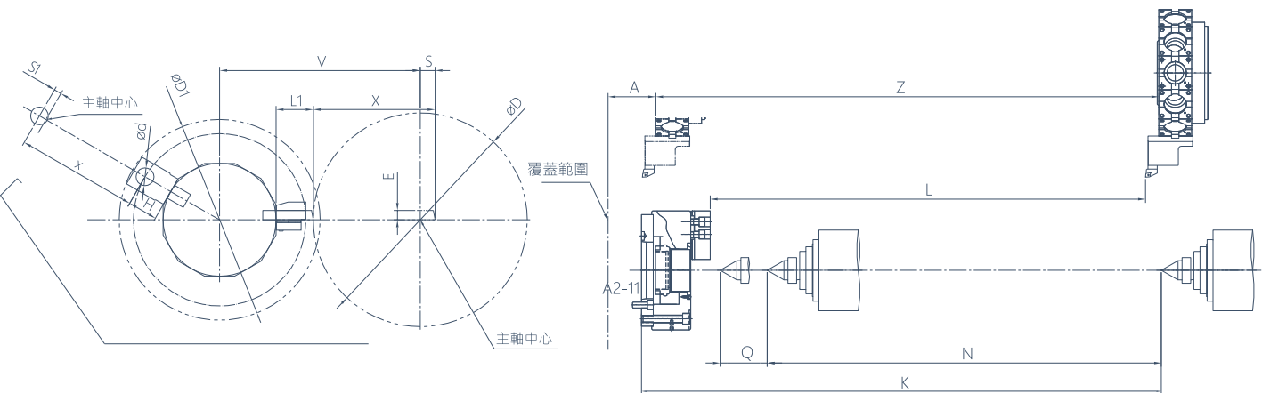
BMT動力刀塔 ( 選配 ) 單位:mm
