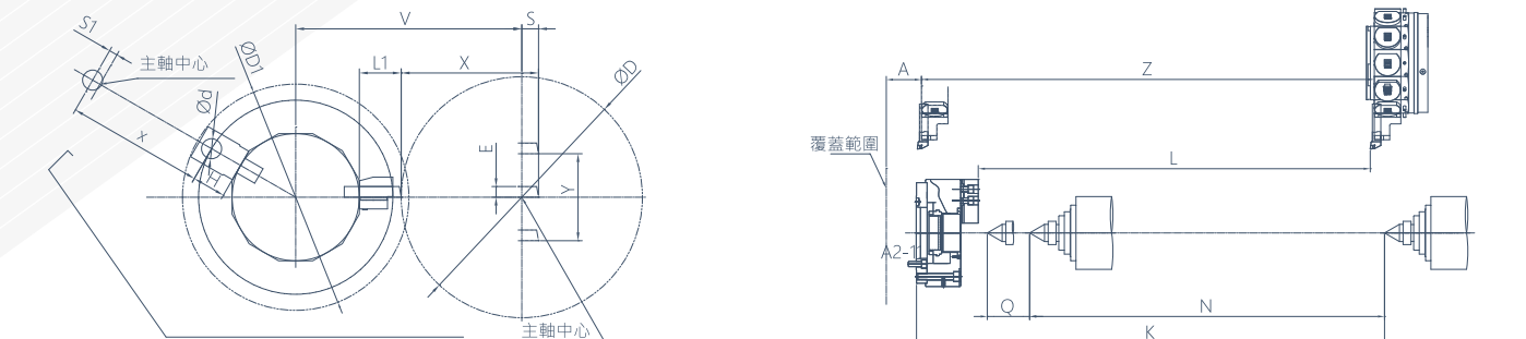
Y軸VDI徑向動力刀塔 ( 選配 ) 單位:mm
